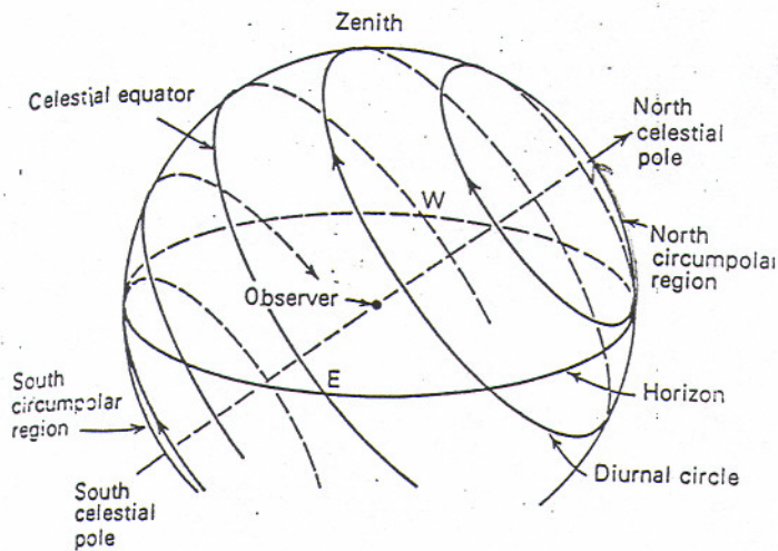
FIG. 7-9 Sky from latitude 34° N.
